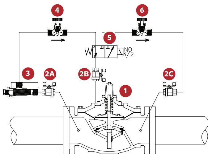
SCHEMATIC A-0593C
